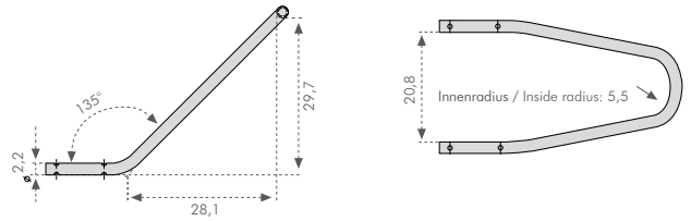
Bemaßung Radhalterbügel (cm) Dimensions of wheel holder (cm)
